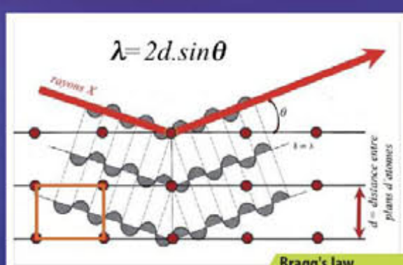
Bragg's law Source : «Voyage dans le Cristal»
